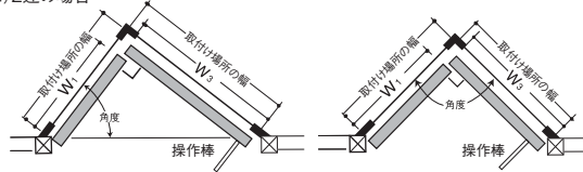
ロ)2連の場合
