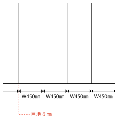
割付図
