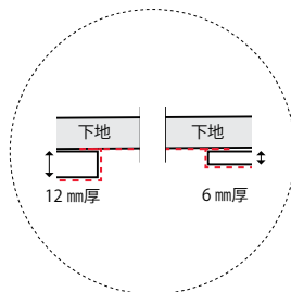
断面拡大図
